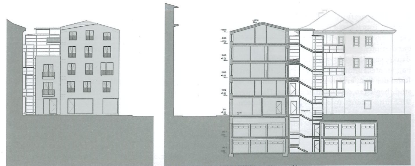
Schnitt A-A
